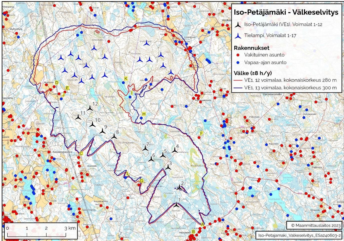
Kuva 11. Varjovälkkeen muodostuminen Iso-Petäjämäen alueella, naapuripuisto huomioiden. Kuvassa on esitetty rajat, joiden sisäpuolella ylitetään maksimisuositus kahdeksan tunnin vuotuisesta varjon välkkeestä.
