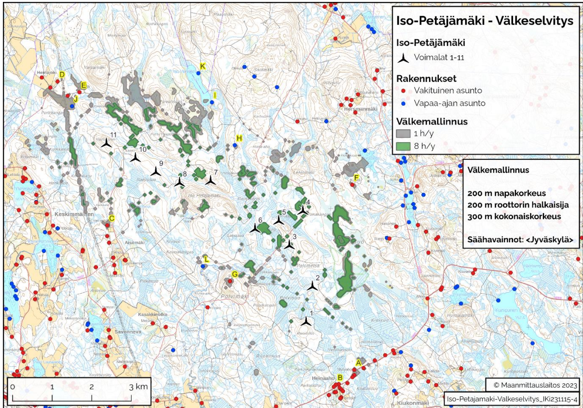
Kuva 7. Varjovälkkeen muodostuminen Iso-Petäjämäen alueella kasvillisuus huomioiden. Havainnointipisteet on merkitty kuvaan (A-L) ja niiden välketasot on esitetty taulukossa 10.
