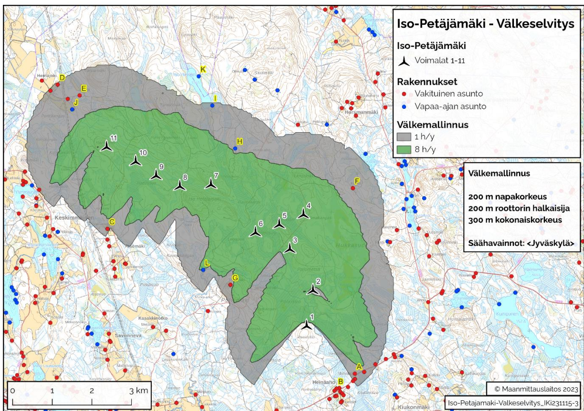
Kuva 4. Varjovälkkeen muodostuminen Iso-Petäjämäen alueella, huomioiden yksinään Iso-Petäjämäki. Havainnointipisteet on merkitty kuvaan (A-L) ja niiden välketasot on esitetty taulukossa 8.
