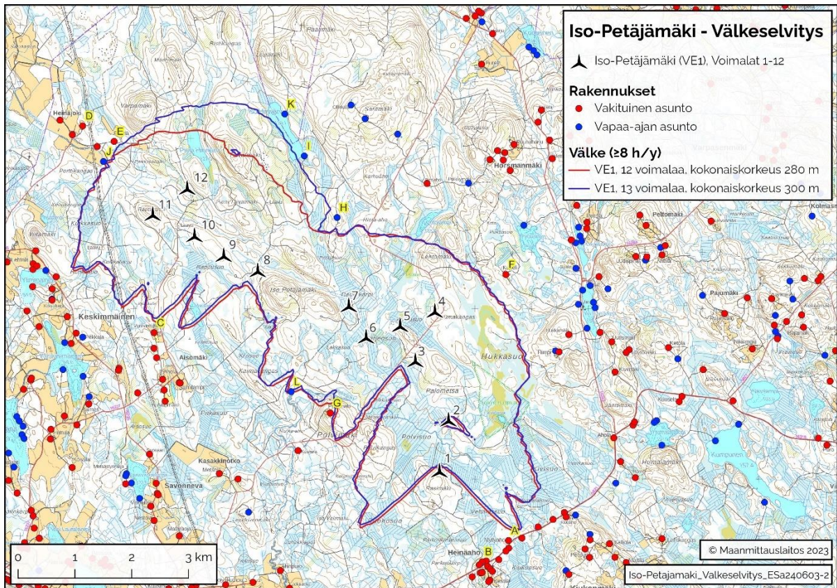
Kuva 10. Varjovälkkeen muodostuminen Iso-Petäjämäen alueella, huomioiden yksinään Iso-Petäjämäki. Kuvassa on esitetty rajat, joiden sisäpuolella ylitetään maksimisuositus kahdeksan tunnin vuotuisesta varjon välkkeestä.
