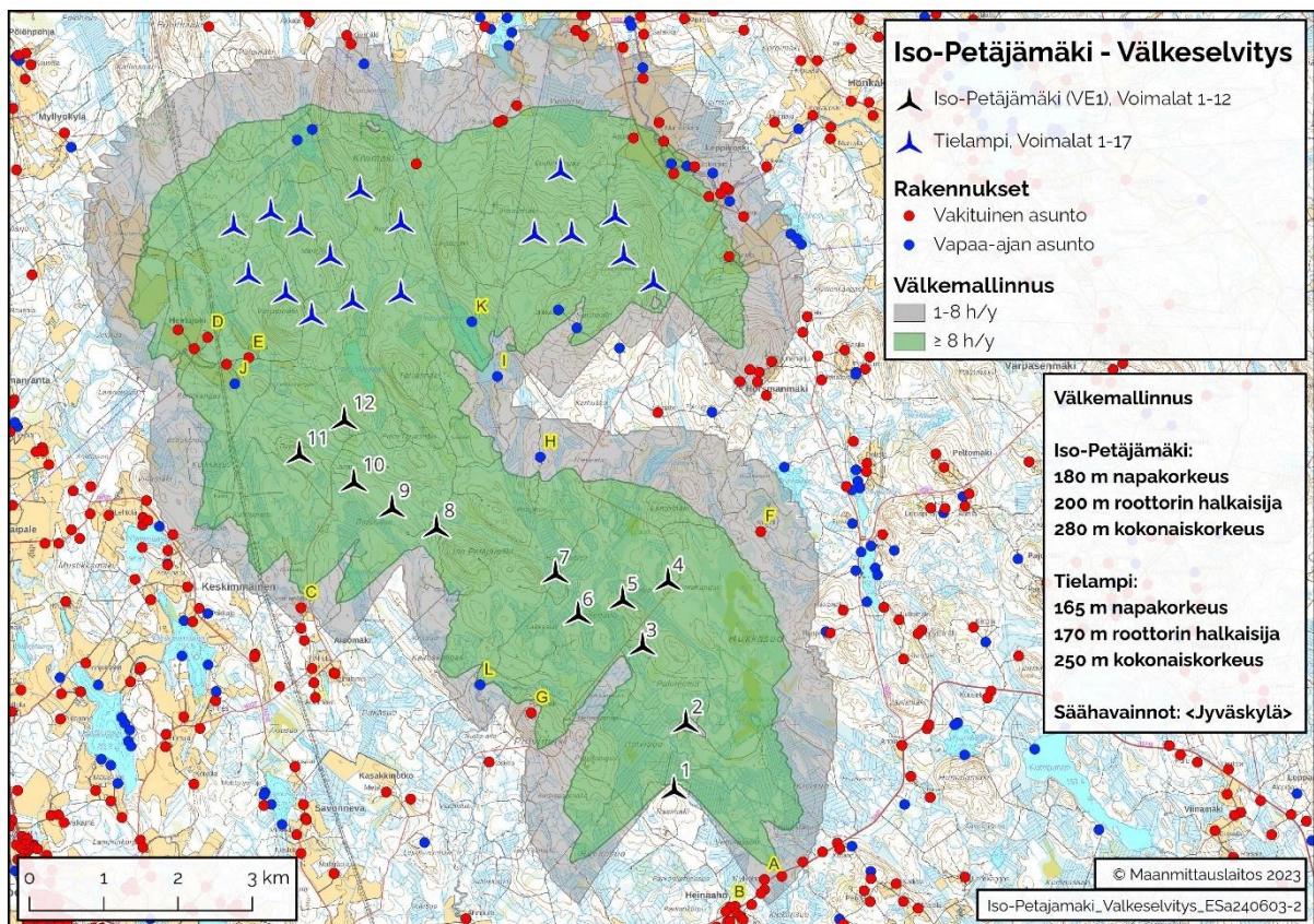
Kuva 8. Varjovälkkeen muodostuminen Iso-Petäjämäen alueella, naapuripuistot huomioiden. Havainnointipisteet on merkitty kuvaan (A-L) ja niiden välketasot on esitetty taulukossa 11.
