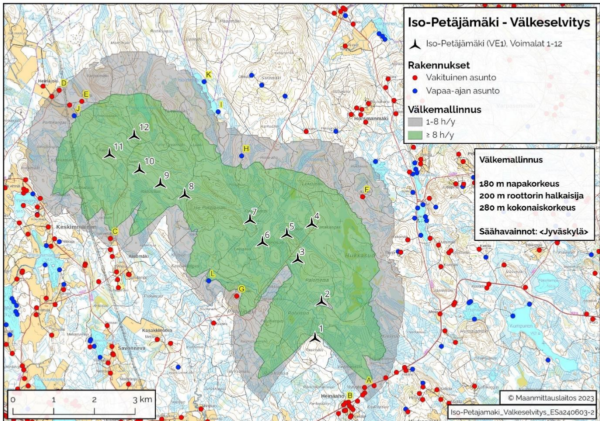
Kuva 2. Varjovälkkeen muodostuminen Iso-Petäjämäen alueella, huomioiden yksinään Iso-Petäjämäki. Havainnointipisteet on merkitty kuvaan (A-L) ja niiden välketasot on esitetty taulukossa 7.
