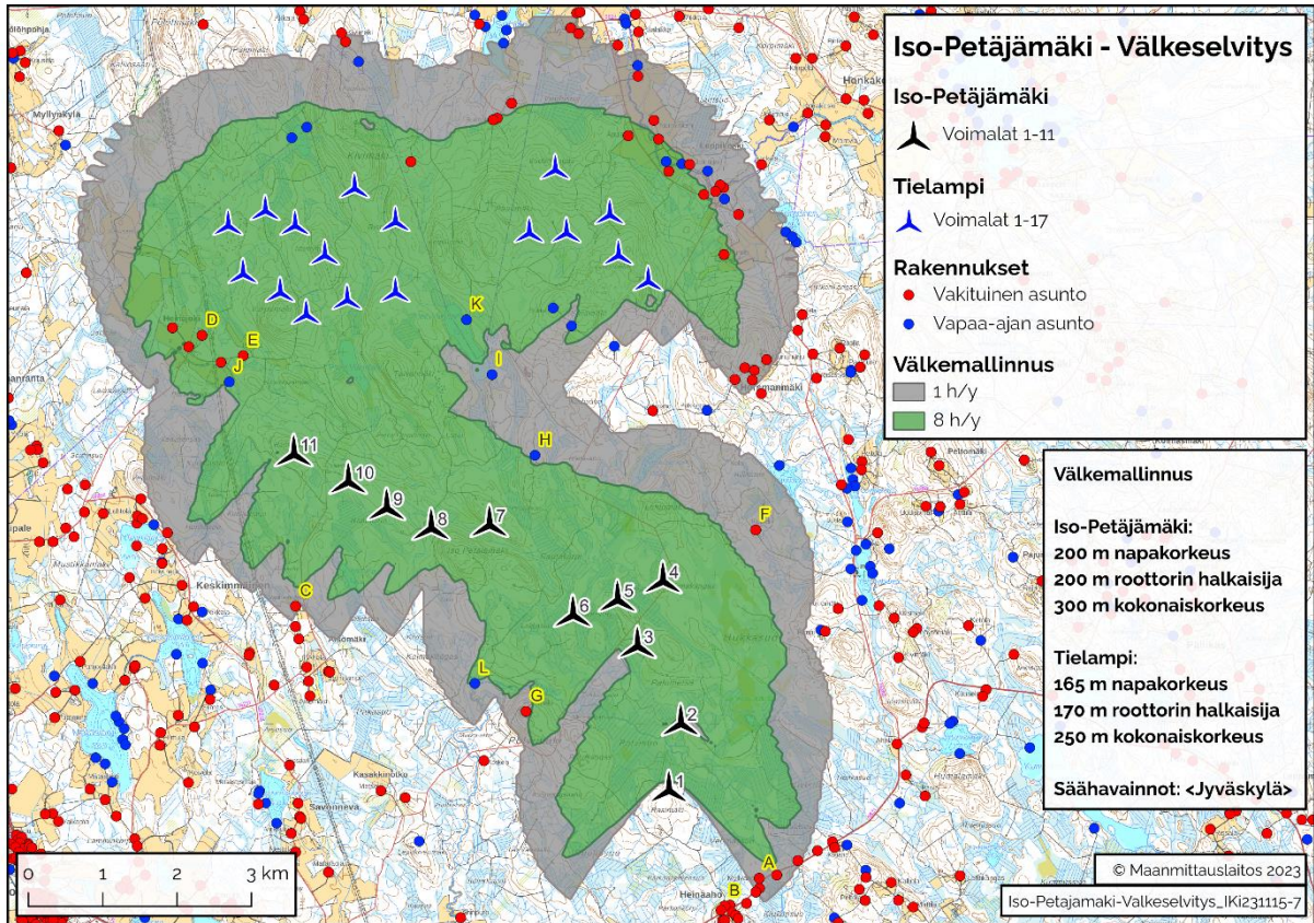
Kuva 9. Varjovälkkeen muodostuminen Iso-Petäjämäen alueella, naapuripuistot huomioiden. Havainnointipisteet on merkitty kuvaan (A-L) ja niiden väketasot on esitetty taulukossa 13.
