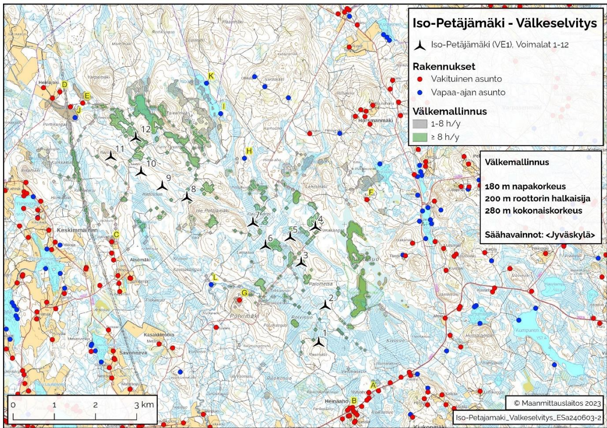
Kuva 6. Varjovälkkeen muodostuminen Iso-Petäjämäen alueella kasvillisuus huomioiden. Havainnointipisteet on merkitty kuvaan (A-L) ja niiden välketasot on esitetty taulukossa 9.
